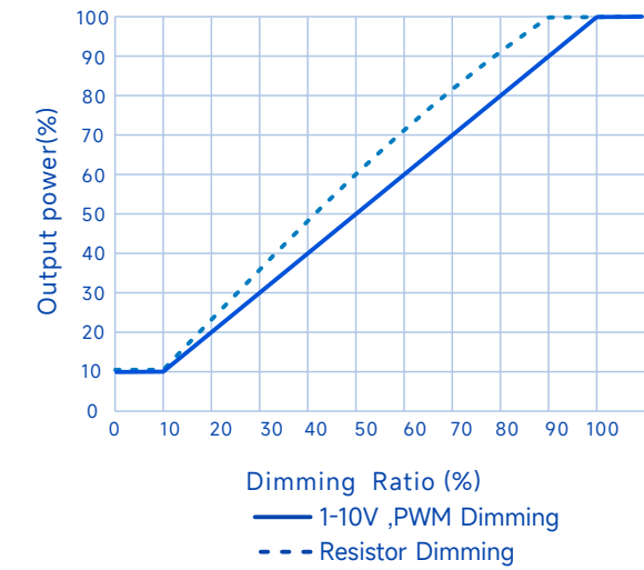
输出功率Vs.调光信号 (BB机型)
